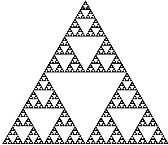
Sierpinski Triangle
